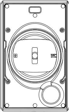
Fig. 1: E6 loudspeaker
